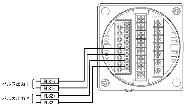
(7) パルス出力2点の場合
