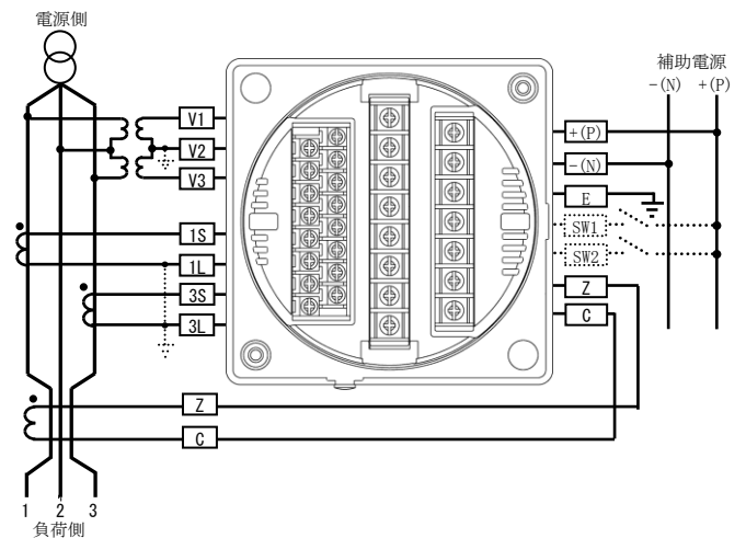
(6) パルス出力+警報出力の場合
