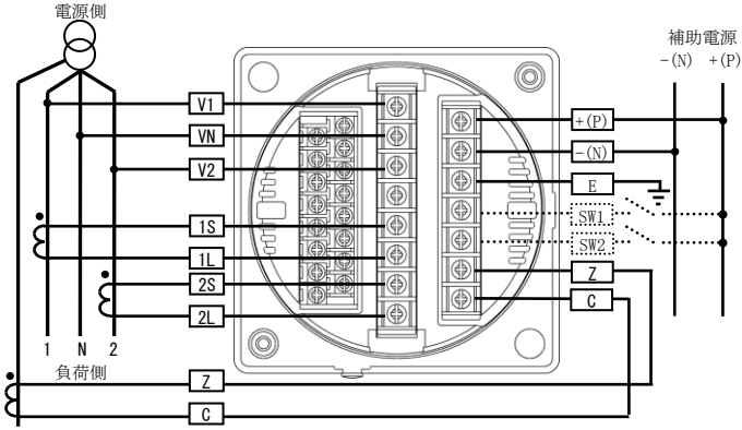
(1) 単相3線式の場合 (※I o rを計算する場合)
