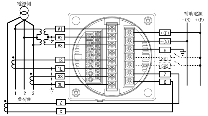
(2) 三相3線式の場合 (※I o rを計算する場合)
