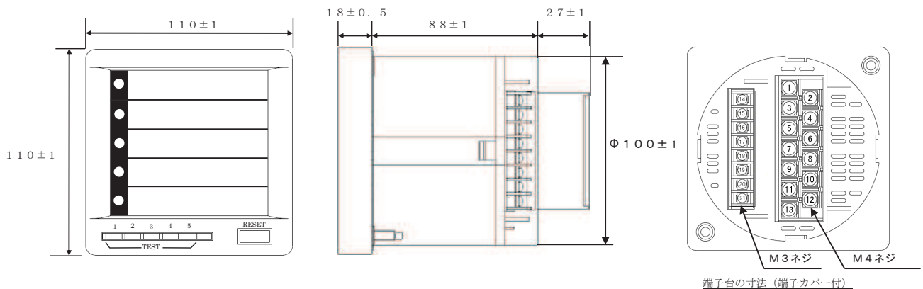
端子台の寸法 (端子カバー付)
