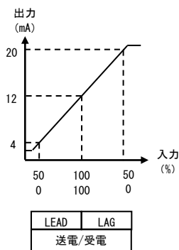
力率
