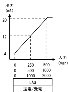
無効電力
