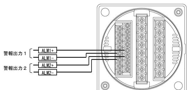
(7) 警報出力2点の場合
