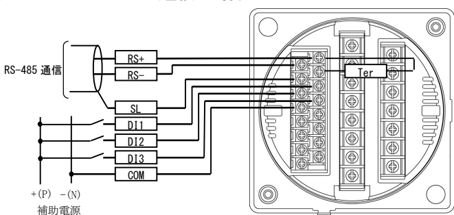
(7) RS-485通信の場合
