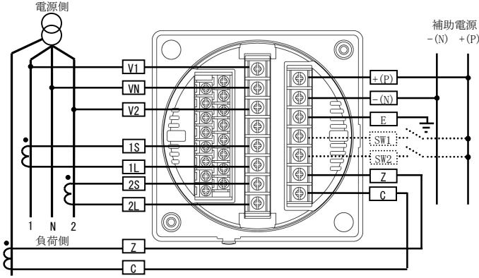
(3) 単相3線式の場合
