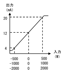
電力 (両振れ)
