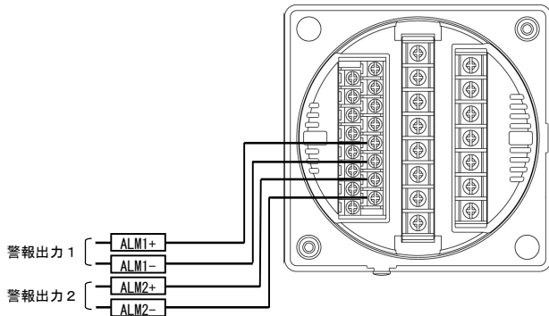
(7) 警報出力 2 点の場合
