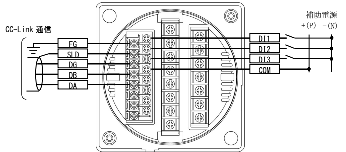
(8) CC-Link 通信の場合
