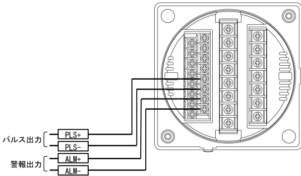
(5) パルス出力+警報出力の場合
