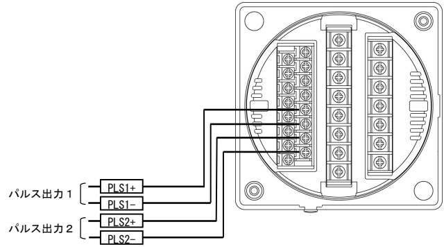
(6) パルス出力 2 点の場合
