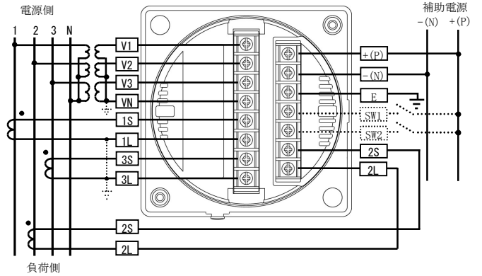
(4) 三相 4 線式の場合
