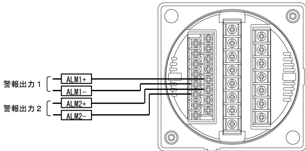
(7) 警報出力2点の場合
