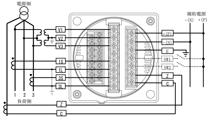
(4) 三相3線式の場合
