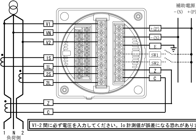
(5) アナログ出力の場合
