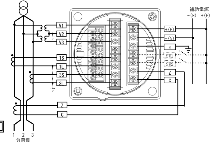
(6) パルス出力+警報出力の場合
