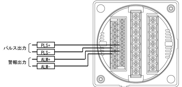
(6) パルス出力+警報出力の場合
