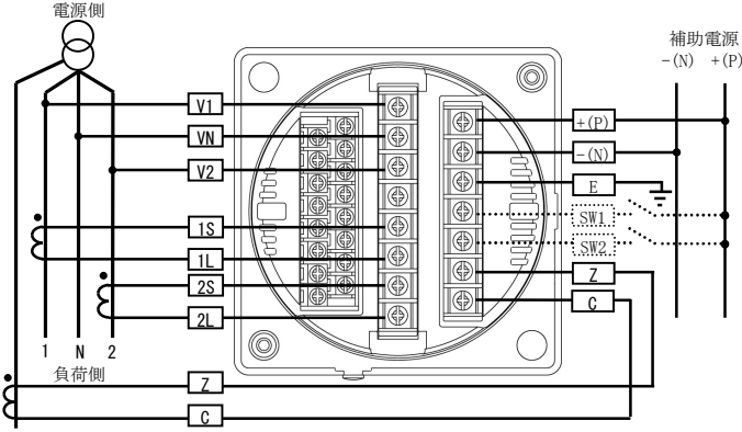
(3) 単相3線式の場合
