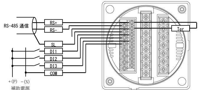
(8) RS-485通信の場合
