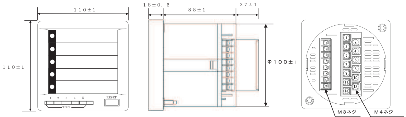
端子台の寸法（端子カバー付）
