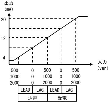
無効電力 (潮流補正)
