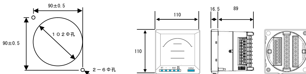
盤穴あけ寸法 (正面から見た図)
