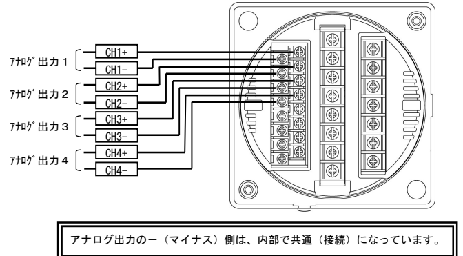
(4) アナログ出力の場合
