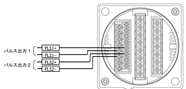
(8) パルス出力2点の場合
