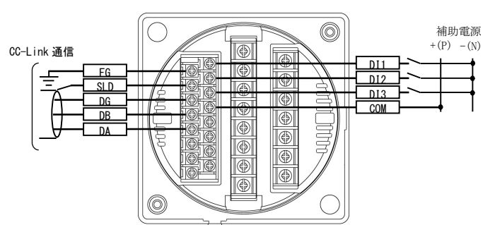
(6) CC-Link通信の場合
