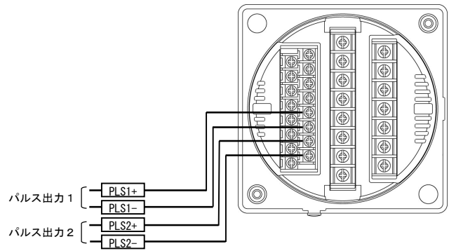
(4) パルス出力2点の場合
