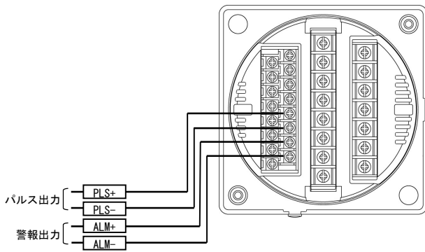
(3) パルス出力+警報出力の場合
