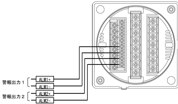
(5) 警報出力2点の場合
