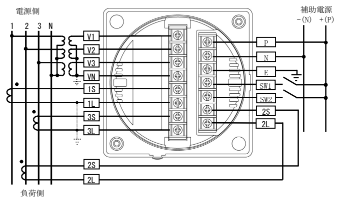
(2) 三相4線式の場合
