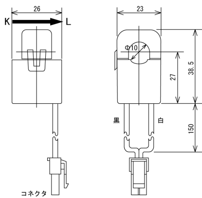
専用クランプCT (CTL-10-CLS35 定格電流5A用)
