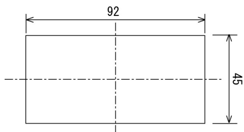
取付寸法図 (単位 : mm)
