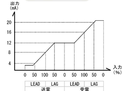
力率 (潮流補正2)
