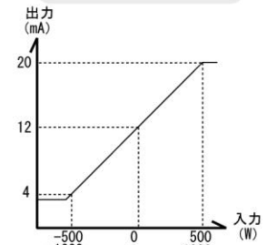
電力 (両振れ)
