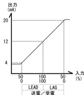
力率
