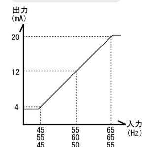
周波数
