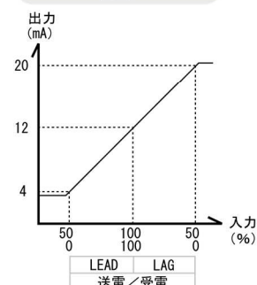
力率
