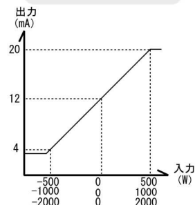
電力 (両振れ)
