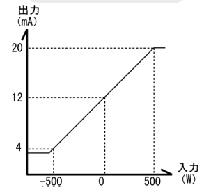
電力 (両振れ)
