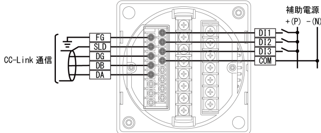
(21) CC-Link 通信の場合
