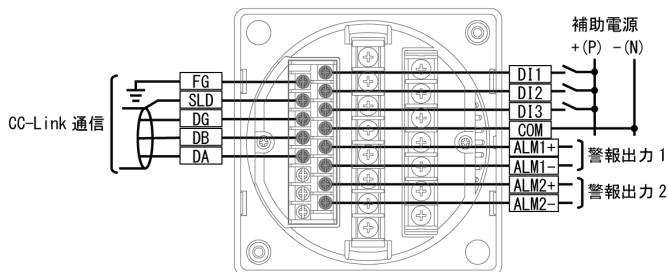
(23) CC-Link 通信の場合+警報出力 2 点
