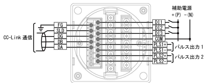
(24) CC-Link 通信+パルス出力 2 点の場合
