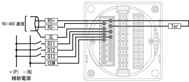
(17) RS-485 通信の場合
