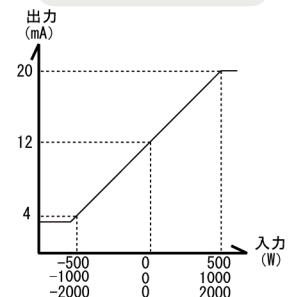
電力 (両振れ)
