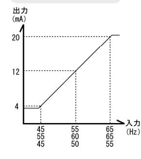
周波数
