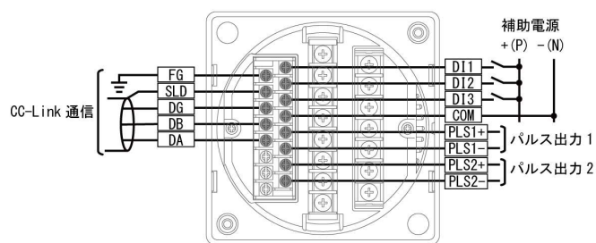
(24) CC-Link 通信+パルス出力 2 点の場合
