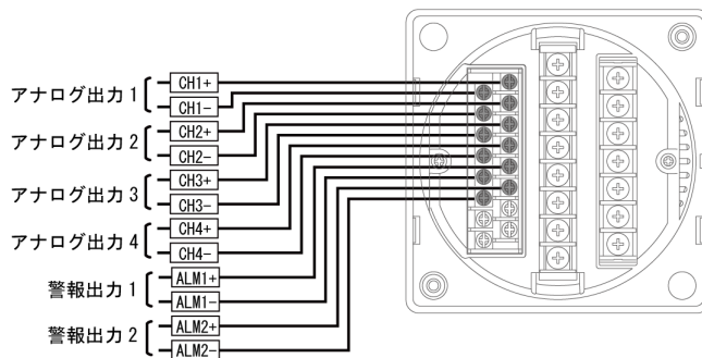
(11) アナログ出力 4 チャンネル+警報 2 点出力の場合
