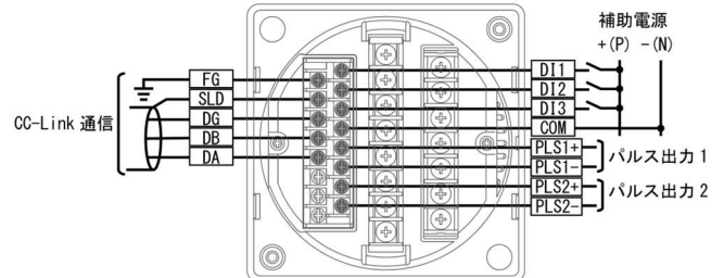
(24) CC-Link 通信+パルス出力 2 点の場合
