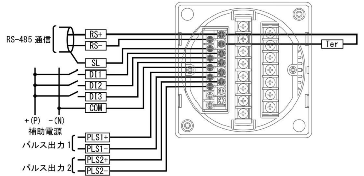
(20) RS-485 通信+パルス出力 2 点の場合
