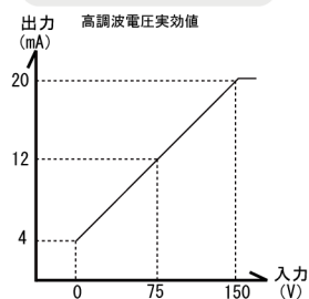
電圧
