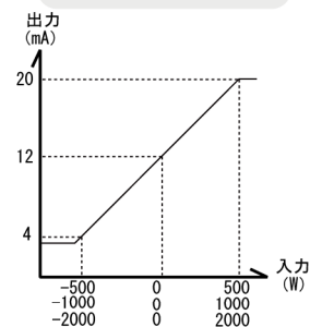
電力 (両振れ)
